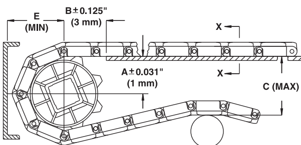
Drive sprocket
