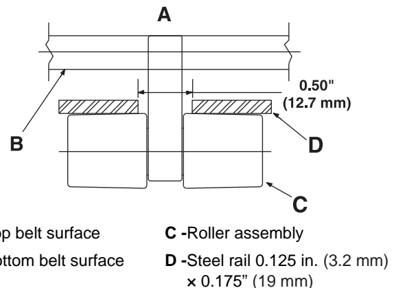
Fig. 3-23 Hold down roller
